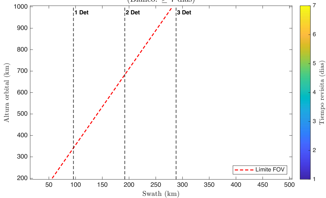
Tiempo Revisita - 1 Satelite(s); 2 Telescopio(s): TMA; Detector 1 (Blanco: \geq 7 dias)
